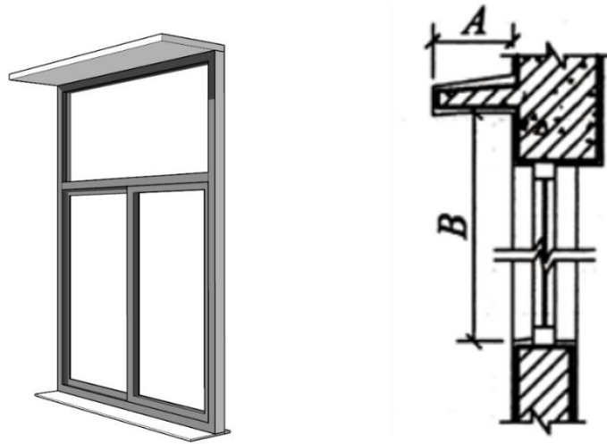
图 B.0.1-1 水平式外遮阳的特征值
