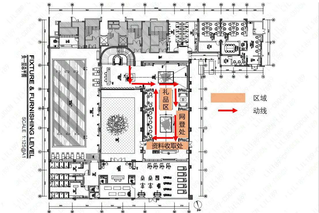
附件 1：资格核验现场布置图
