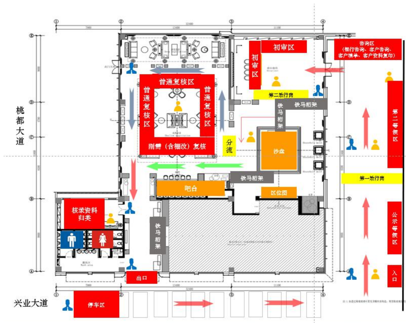
附件 1：资格核验现场布置图
