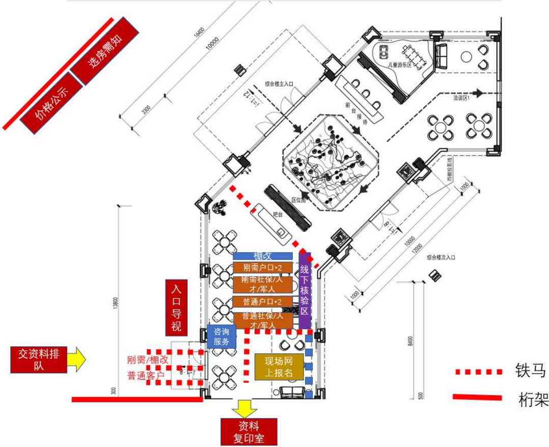
附件 1：资格核验现场布置图
